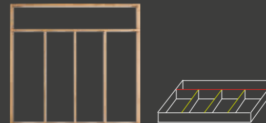
Typ U3: Höhe 52 mm oder 92 mm Tiefe 340 - 520 mm / Breite 350 - 650 mm
