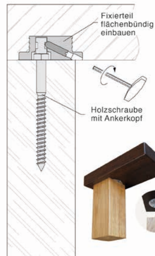
Universalverbinder
