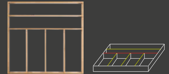
Typ U5: Höhe 52 mm oder 92 mm Tiefe 340 - 550 mm / Breite 350 - 650 mm
