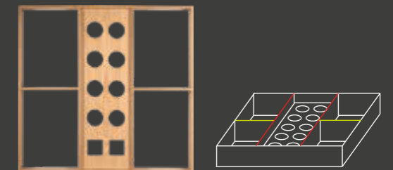
Typ U6: Höhe 52 mm oder 92 mm Tiefe 340 - 550 mm / Breite 500 - 650 mm inkl. quadratischer Fächer für Salz- und Pfefferstreuer
