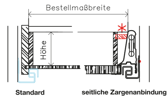
Detailskizze: Zargenanbindung
